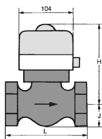
1020 taraudé
