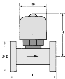
1020 à brides
